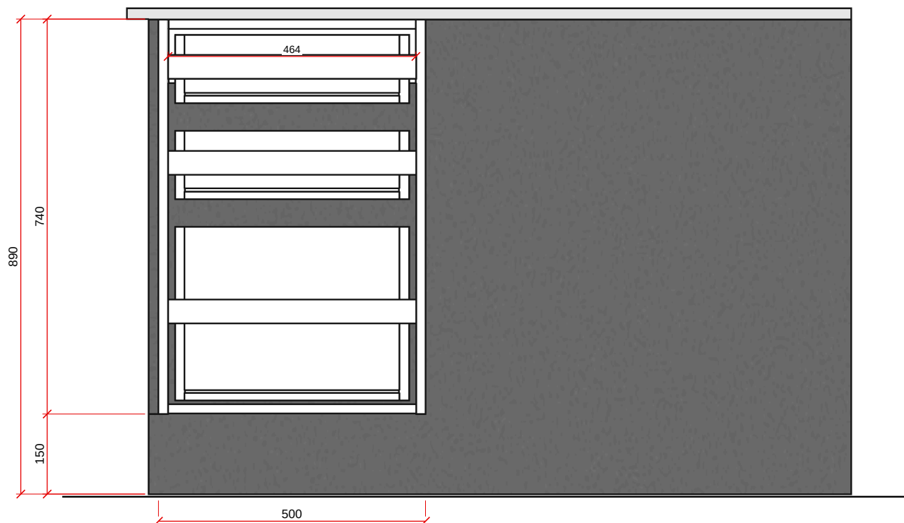
VISTA B - ESC. 1:10
